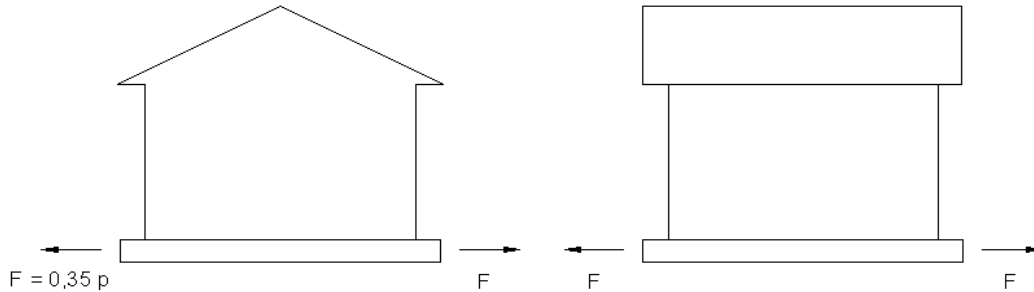
Efforts horizontaux dans les fondations
