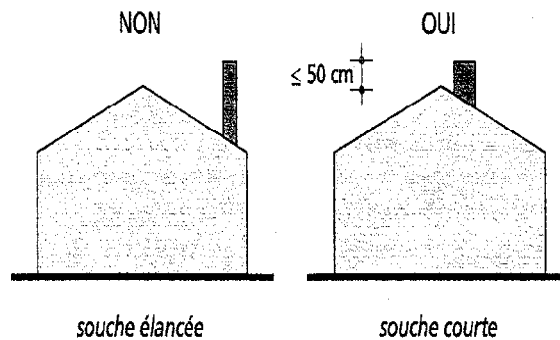
Conduits de fumée.
